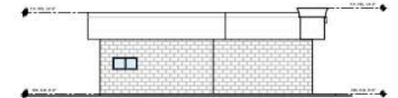
5 EXISTING LEFT ELEVATION Scale: 1/8" = 1'-0"
